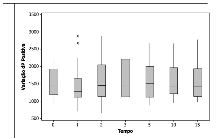
Figura 15: Box-plot da dP/dt por Tempo.
