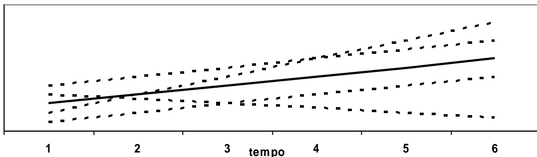
Figura 2: Evolução de uma determinada variável ao longo da resposta (eixo Y); inclinações e interceptos diferentes para indivíduos diferentes (linha tracejada = indivíduos, linha contínua = população).
